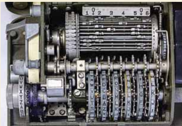
ПОРТАТИВНАЯ МЕХАНИЧЕСКАЯ ШИФРОВАЛЬНАЯ МАШИНА М-209 ВЫПУСКАЛАСЬ В США ПО ЛИЦЕНЗИИ
